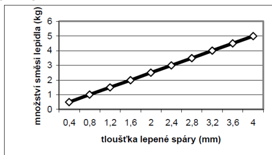
Spotřeba směsi lepidla v závislosti na tloušťce lepené spáry na 1m 2 plochy
